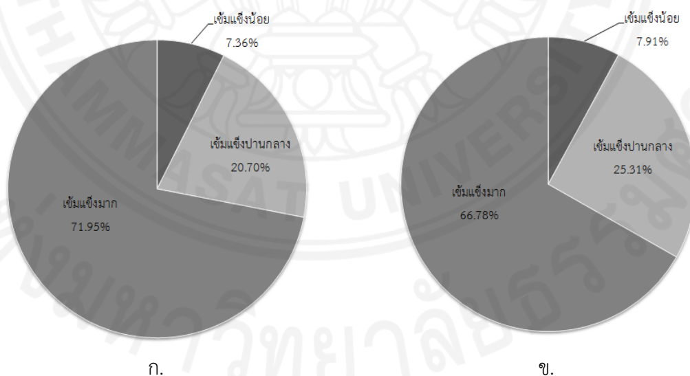
ภาพที่ 4.2 ร้อยละของขนาดหรือจำนวนครอบครัว ในแต่ละระดับความเข้มแข็งของครอบครัว ในปี พ.ศ. 2555 (ก.) และ พ.ศ. 2556 (ข.) กรณีข้อมูลเชิงกลุ่ม (ข้อมูลเดิม) โดยการวิเคราะห์แบ่งกลุ่มด้วยวิธี k-modes
