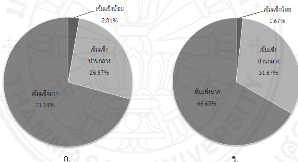
ภาพที่ 4.1 ร้อยละของขนาดหรือจำนวนครอบครัว ในแต่ละระดับความเข้มแข็งของครอบครัว ในปี พ.ศ. 2555 (ก.) และ พ.ศ. 2556 (ข.) โดยการวิเคราะห์แบ่งกลุ่มด้วยวิธี k-means
