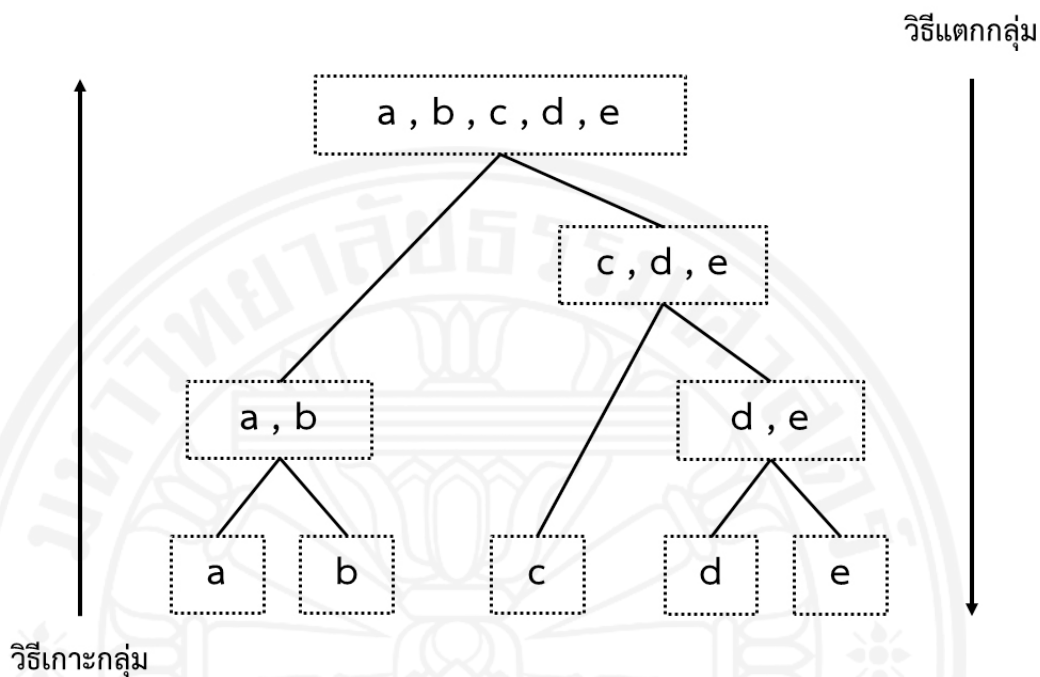
ภาพที่ 2.1 แผนภาพแสดงการวิเคราะห์แบ่งกลุ่มแบบมีขั้นตอน ด้วยวิธีการเกาะกลุ่ม และวิธีการแตกกลุ่ม
