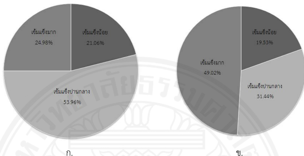
ภาพที่ 4.3 ร้อยละของขนาดหรือจำนวนครอบครัว ในแต่ละระดับความเข้มแข็งของครอบครัว ในปี พ.ศ. 2555 (ก.) และ พ.ศ. 2556 (ข.) กรณีข้อมูลทวิภาค (ข้อมูลที่แปลง) โดยการวิเคราะห์แบ่งกลุ่มด้วยวิธี k-modes
